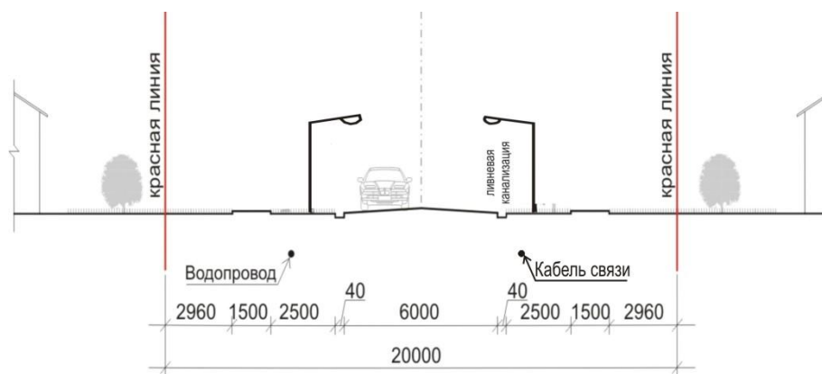
Рис.1 Поперечный профиль главной улицы Ключевой М 1:200
