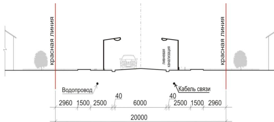
Рис.4 Поперечный профиль главной улицы Ключевой М 1:200
